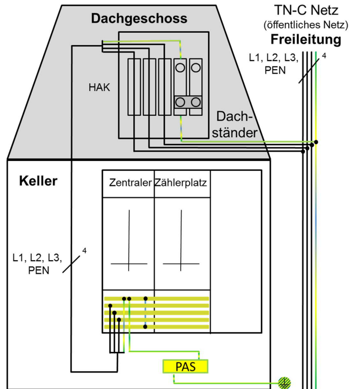
Abbildung D.1 Beispiel für einen Freileitungsnetzanschluss
